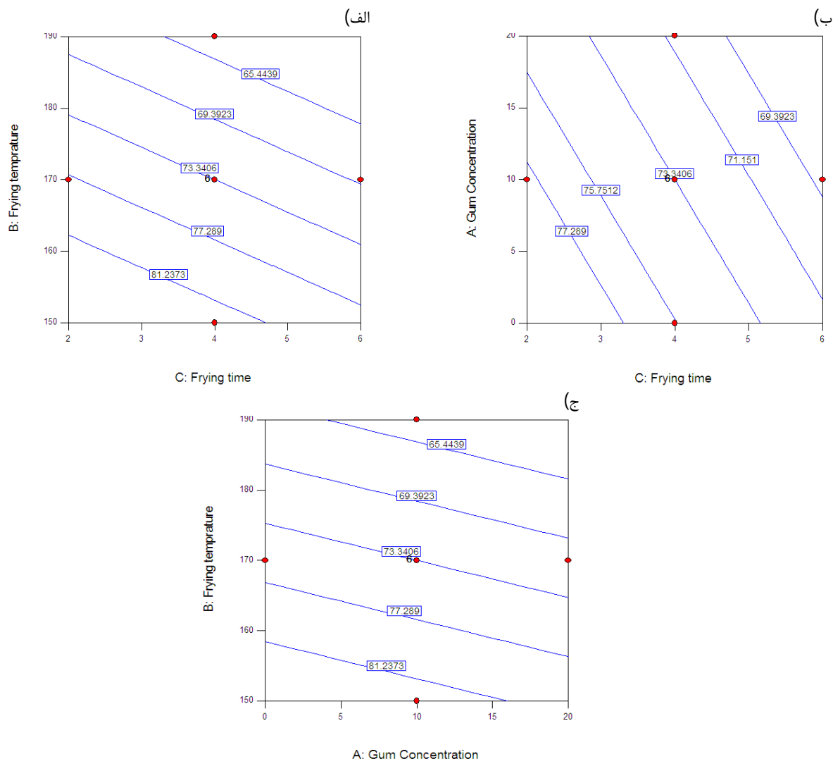
شکل 1. تغییرات میزان رطوبت نمونه‌های چیپس هویج سرخ شده تحت تأثیر الف- غلظت ژل آلوه‌ورا و زمان سرخ کردن (دمای سرخ کردن 170 درجه سلسیوس) ب- دما و زمان سرخ کردن (غلظت ژل آلوه‌ورا 10%) و ج- غلظت ژل آلوه‌ورا و دمای سرخ کردن (زمان سرخ کردن 4 دقیقه)
