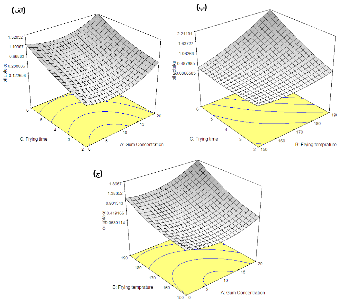
شکل 2. تغییرات میزان جذب روغن نمونه‌های چیپس هویج سرخ شده تحت تأثیر الف- غلظت ژل آلوه‌ورا و زمان سرخ کردن (دمای سرخ کردن 170 درجه سلسیوس) ب- دما و زمان سرخ کردن (غلظت ژل آلوه‌ورا 10%) و ج- غلظت ژل آلوه‌ورا و دمای سرخ کردن (زمان سرخ کردن 4 دقیقه)
