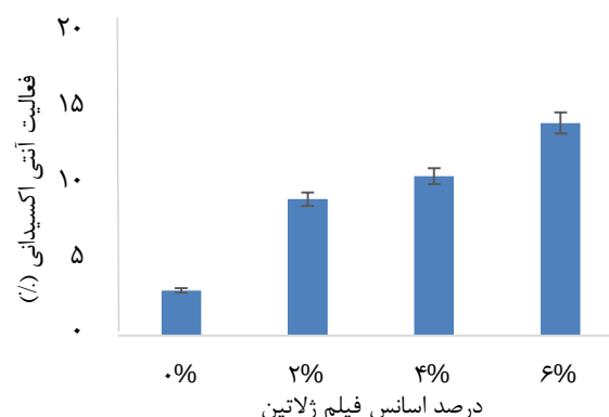
شکل ۱. فعالیت آنتی اکسیدانی فیلم ژلاتین حاوی اسانس کندر
