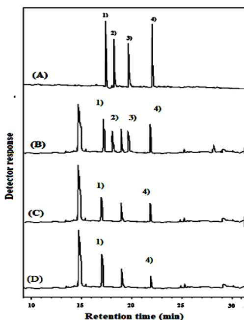
شکل ۳. کروماتوگرام‌های GC-FID محلول استاندارد فیتواسترول‌ها به غلظت ۲۵۰ میلی گرم بر کیلوگرم در استون (نسبت به هریک از آنالیت‌ها (A)، نمونه خامه اسپایک شده با غلظت ۰/۵ میلی گرم بر لیتر از هر یک از آنالیت‌ها
