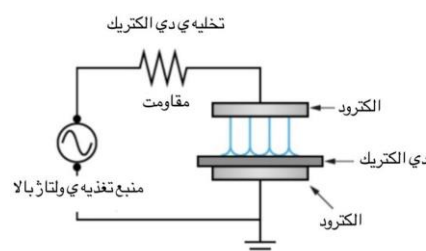
شکل ۲. تصویر شماتیک و اصلی فرایند تخلیه سد دی الکتریک. عمل پلاسما DBD در حالت رشته‌ای
