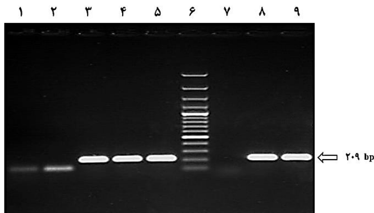
شکل ۱. تصویر ژل آگارز ۱/۵ درصد (Invitrogen, G501802) محصولات PCR جدایه‌های پنیر موتال با آغازگر اختصاصی جنس لاکتوباسیلوس. ستون ۶: مارکر (Fermentas SN 0623, Germany) ۱۰۰bp، ستون ۵: کنترل مثبت حاوی DNA باکتری لاکتوباسیلوس پلانتاروم (PTCC 1058)، ستون ۷: کنترل منفی بدون DNA الگو، ستون‌های ۱ تا ۴ و ستون‌های ۸ و ۹: نمونه‌های جداسازی شده از پنیر.
