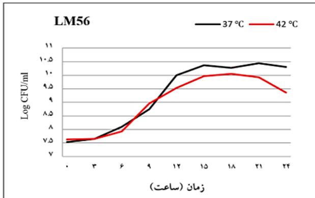
شکل ۲. نمودار رشد باکتری‌های لاکتوباسیلوس منتخب جدا شده از پنیر موتال
