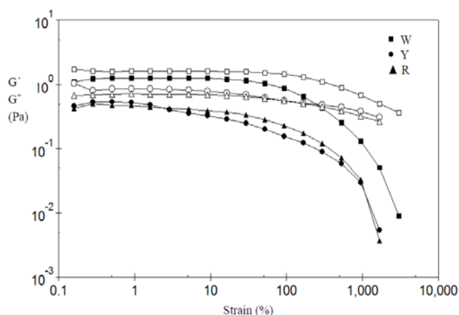
شکل ۲. منحنی تغییرات مدول ذخیره در روبش کرنش، فرکانس ۱ Hz سه نوع صمغ زرد (اشکال توخالی G' و توپر G'' )
